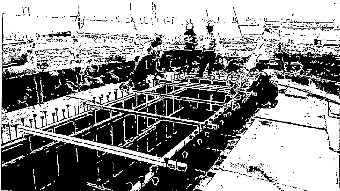
ENCOFRADO DE CISTERNA
